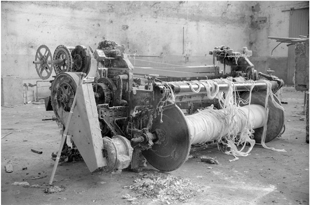
Face arrière du métier à tisser. Moteur Alsthom au premier plan, à gauche de l'ensouple.
