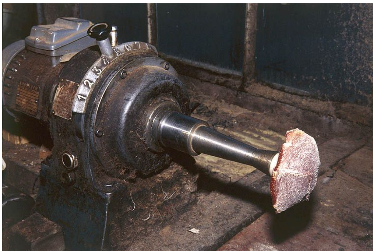
Vue rapprochée : variateur et disque de polissage.
