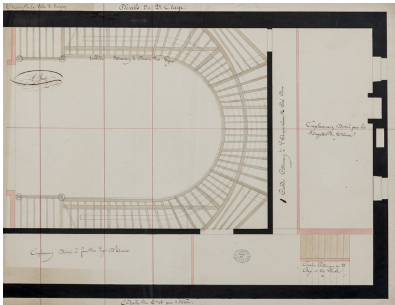
Construction de la salle de spectacle. Détail du 2e étage. Pour le charpentier. 1832.
