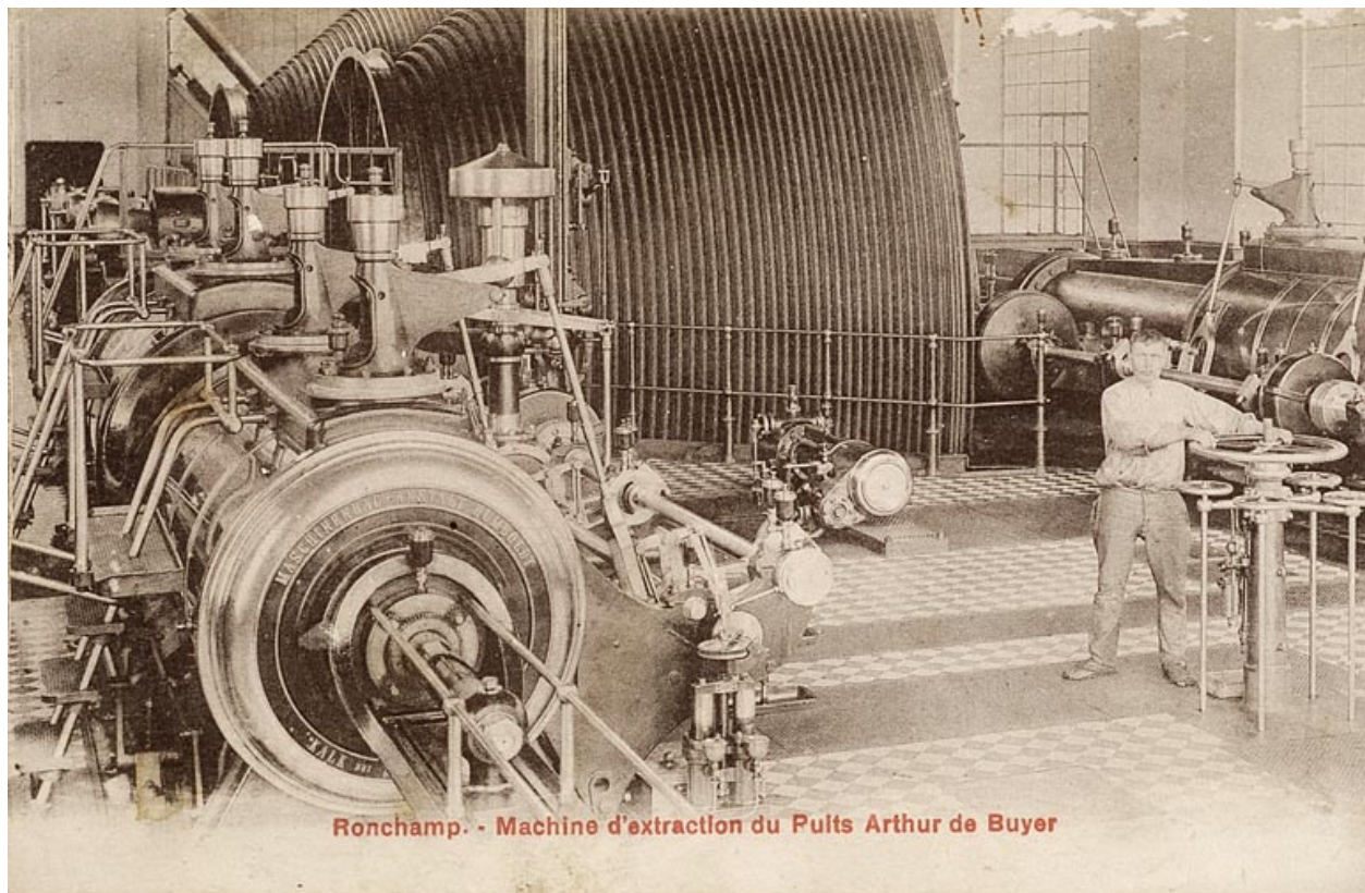
Ronchamp. - Machine d'Extraction du Puits Arthur de Buyer, [avant 1923].
