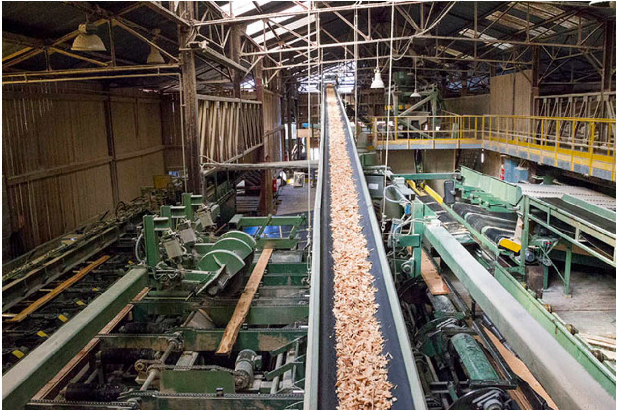
Ateliers de débitage (N et M) : machines de reprise et tapis roulant d'évacuation des sciures et des copeaux.
