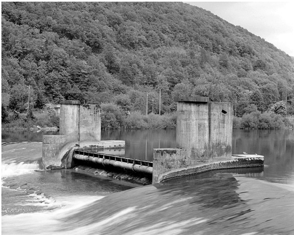
La vanne clapet.
