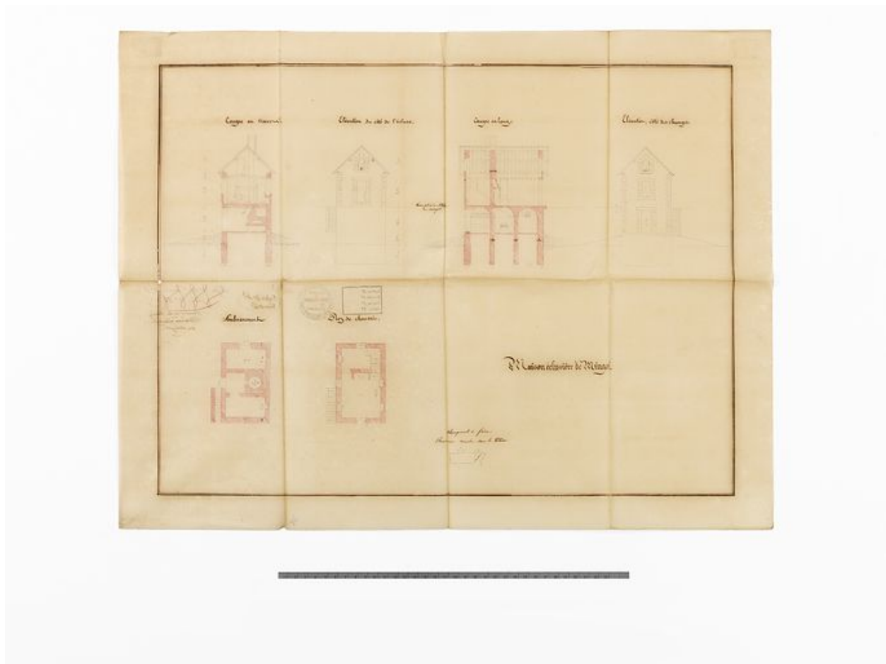
"Maison éclusière de Mingot". Plan, coupe et élévation. (Archives VNF-direction territoriale Centre-Bourgogne ; subdivision de Corbigny)
