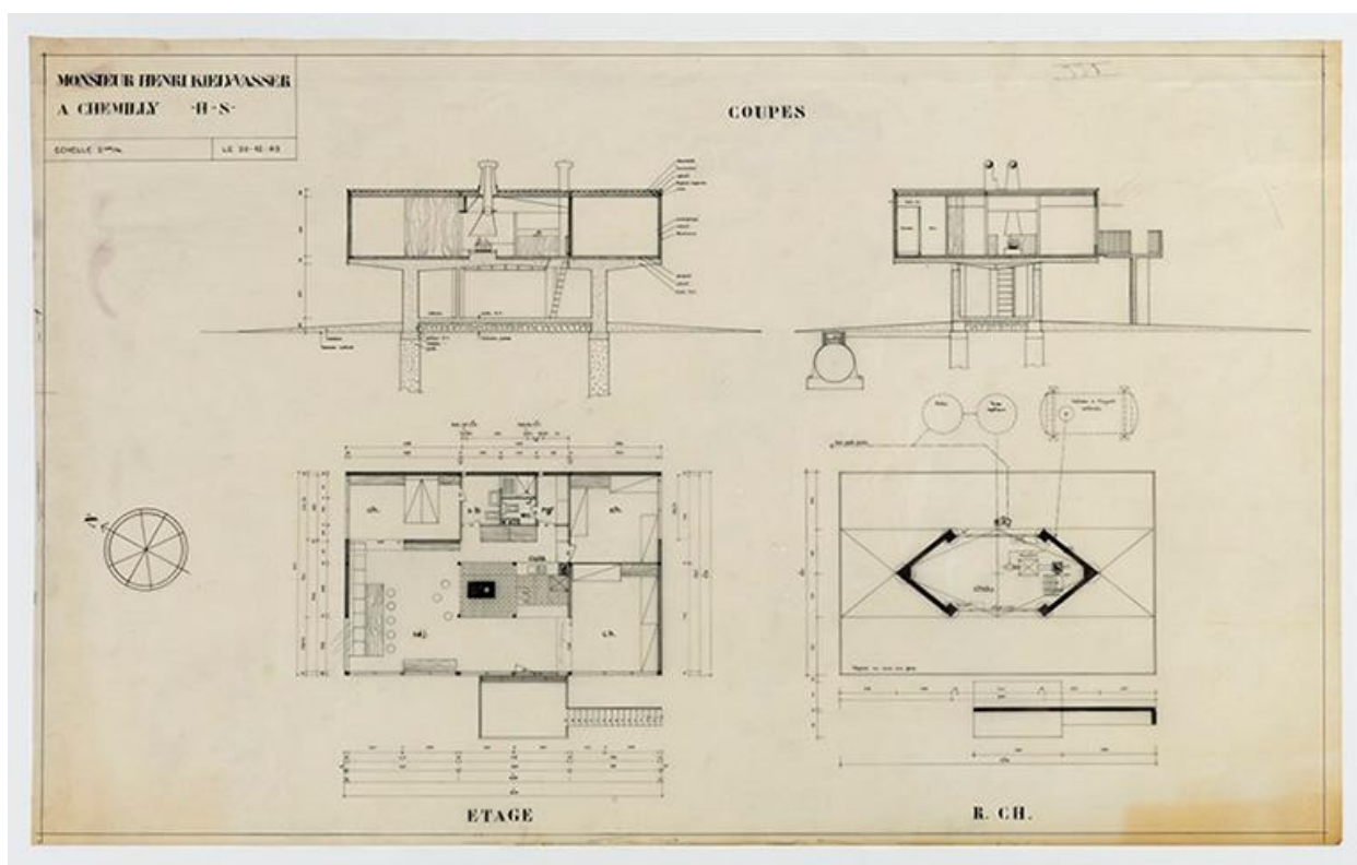
Plans en coupe de la villa.
