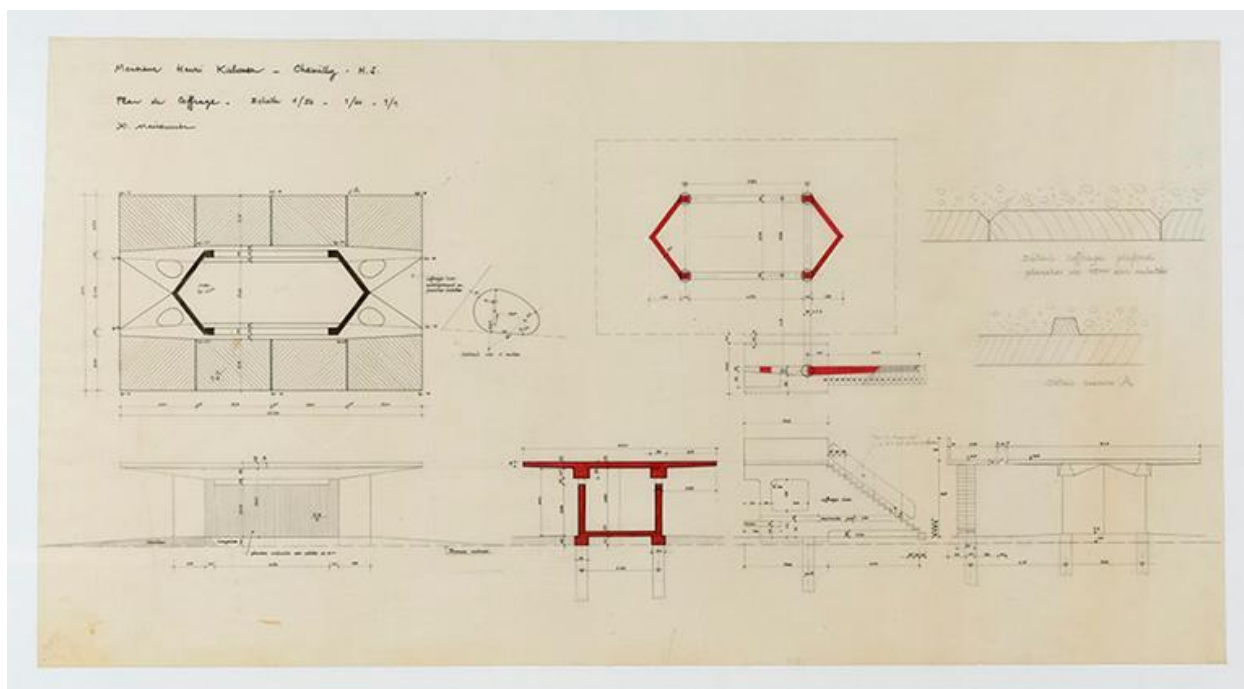
Plan en coupe du coffrage de la pile de la maison
