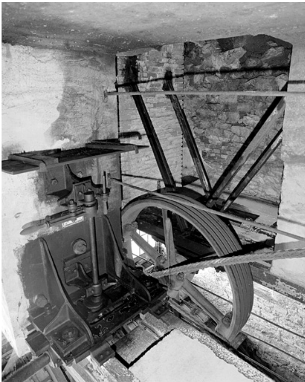
Roue de transmission de la machine à vapeur et système de couplage de la turbine.
