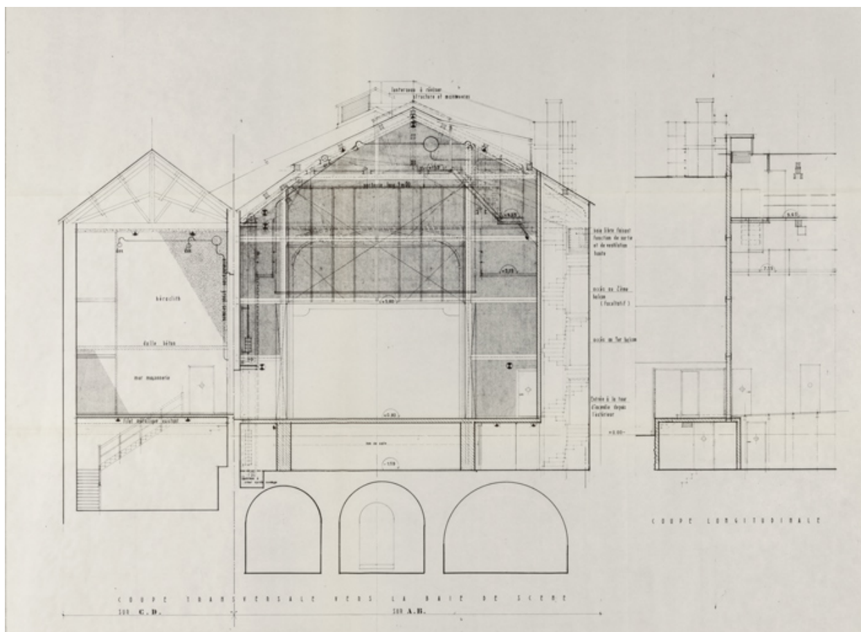
Ville de Nevers. Théâtre municipal. Mise en conformité. 1A. [Détail :] Coupe transversale sur baie de scène. 1976.
