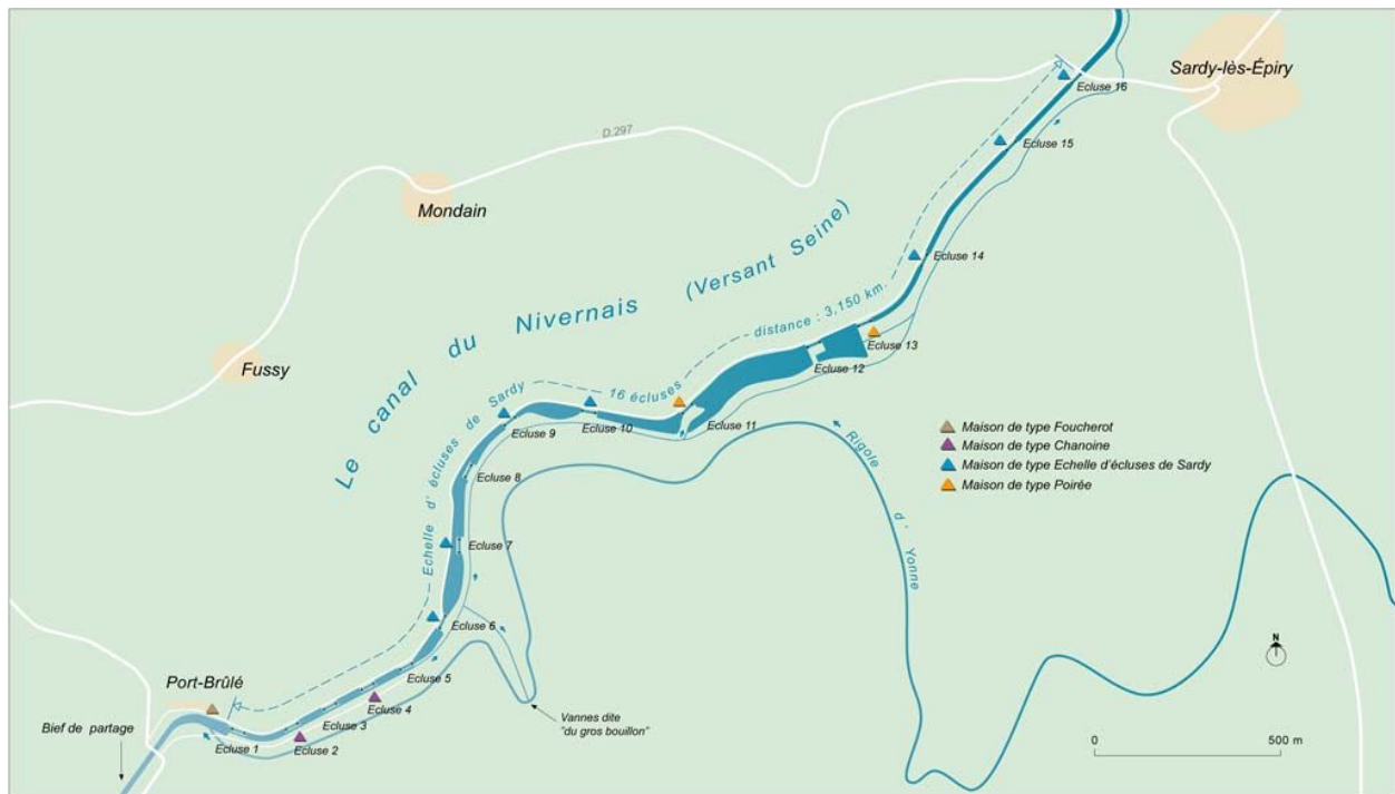
Carte schématique de l'échelle d'écluses de Sardy.
