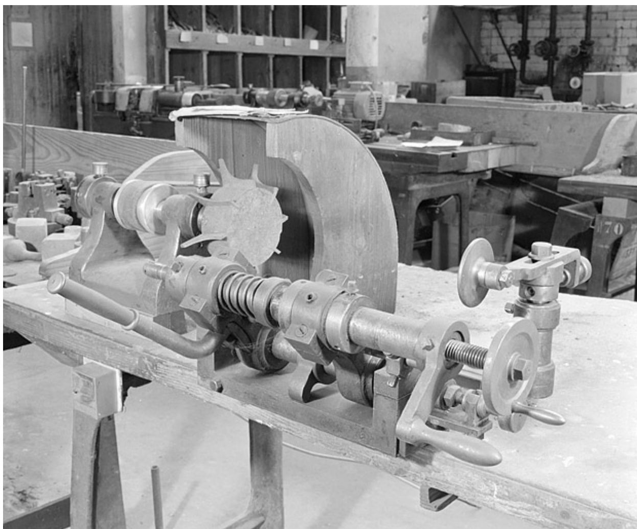
Vue d'ensemble rapprochée de l'arrondisseur (atelier principal).
