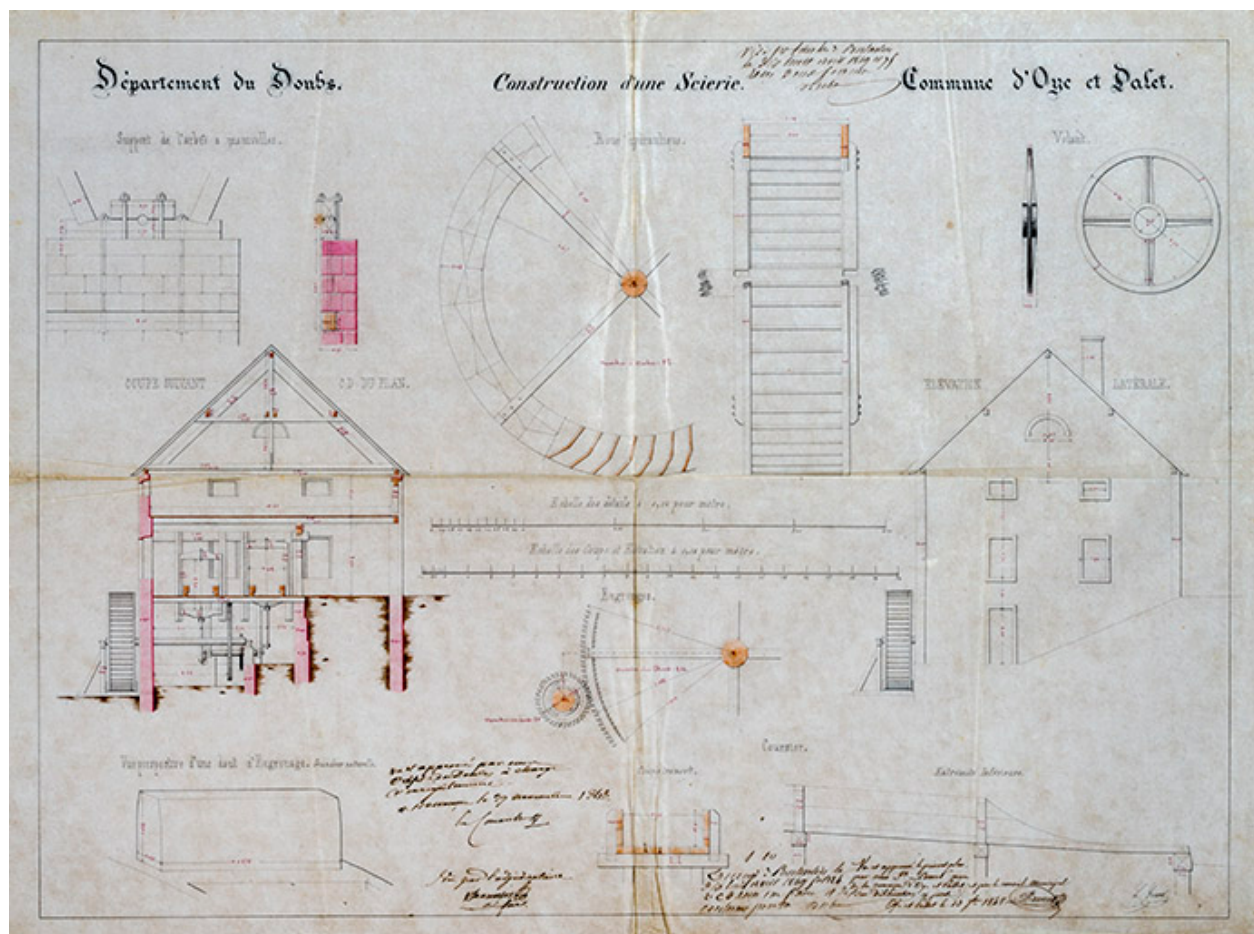
Moulin et scierie communale, Oye-et-Pallet : construction d'une scierie [Élévation, coupe et détails], 1848.
