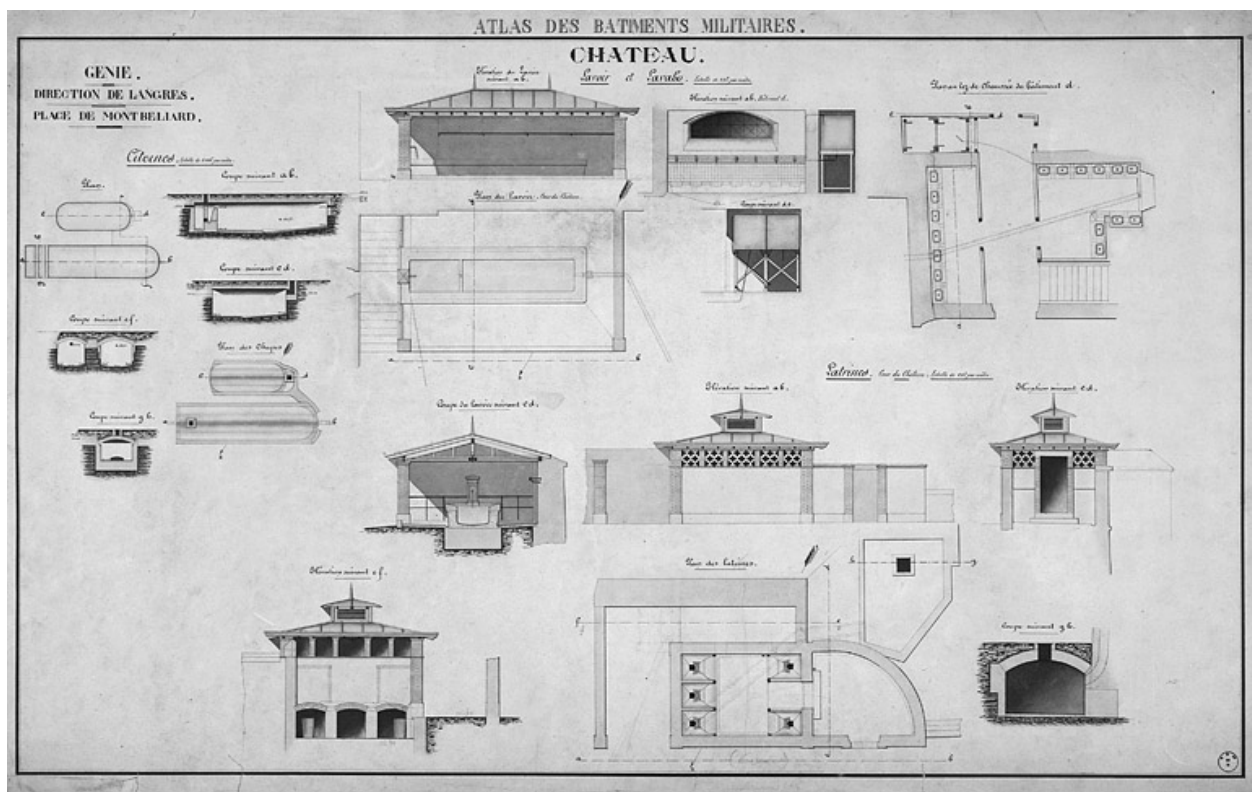
Atlas des bâtiments militaires [...] Feuille 11 [lavoir, lavabo, citernes et latrines], années 1880.
