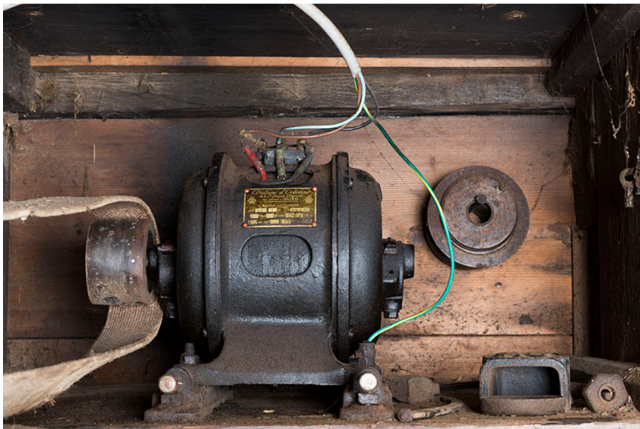
Atelier : moteur de 0,5 ch des Ateliers d'Orléans de la Compagnie générale d'Electricité (type L05 3 PH n° 30532).
