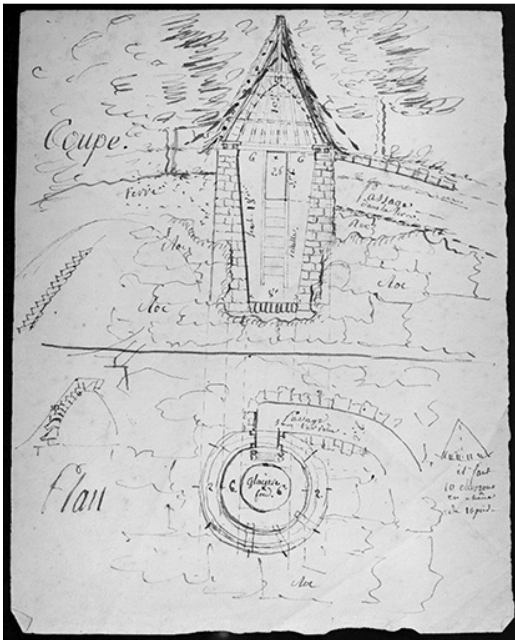
Plan et coupe d'une glacière.
