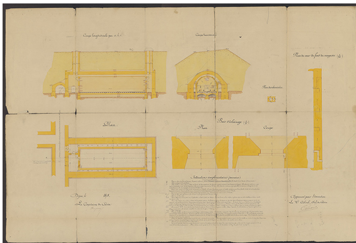
[Plans et coupes du magasin à poudre au fort de Varois]. 1878.
