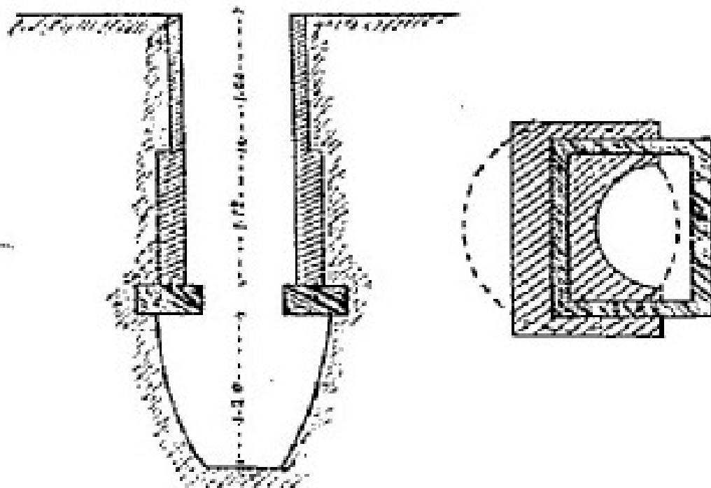
Fig. 63. — COUPE ET PLAN DU CAPTAGE DE LA SOURCE DE MAIZIÈRES.
