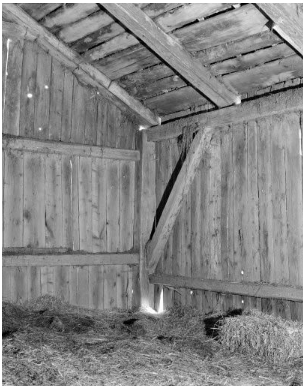
Détail de charpente : angle arrière droit.
