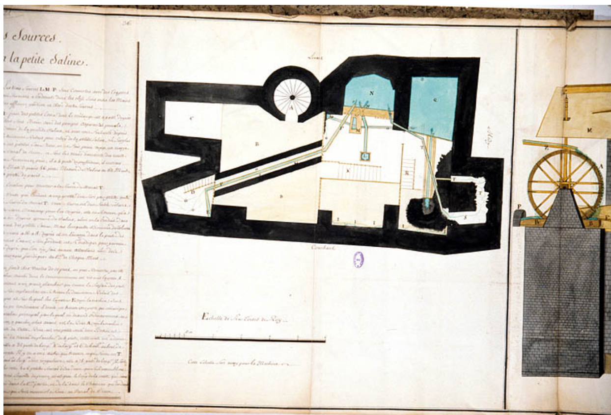
Machines Hydrauliques Qui Elèvent Les Eaux salées et douces du puit à Muire [plan du puits à muire], 1756.
