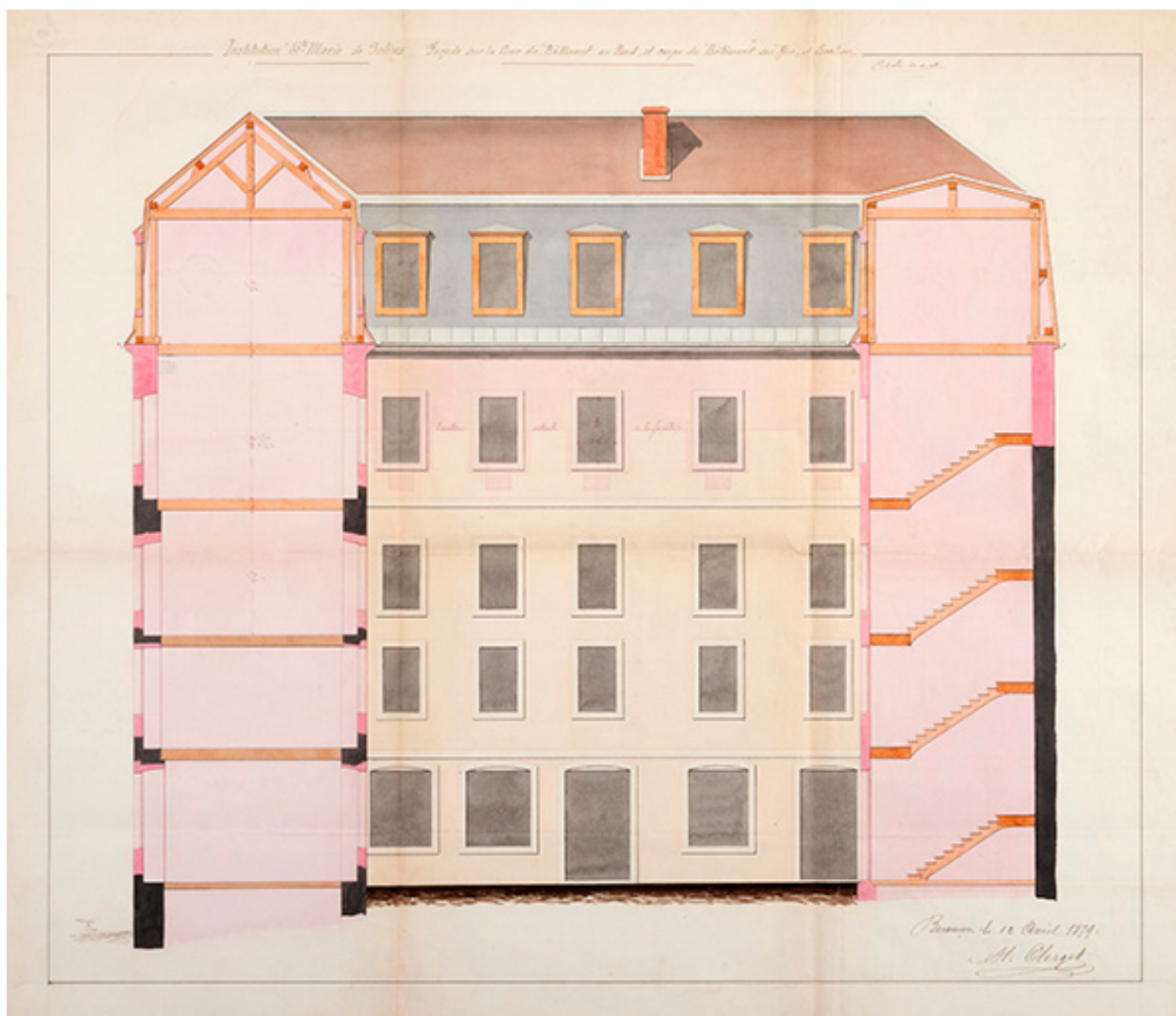
Institution Sainte-Marie de Salins. Façade sur la cour du bâtiment au nord, et coupe du bâtiment sur rue, 1879.
