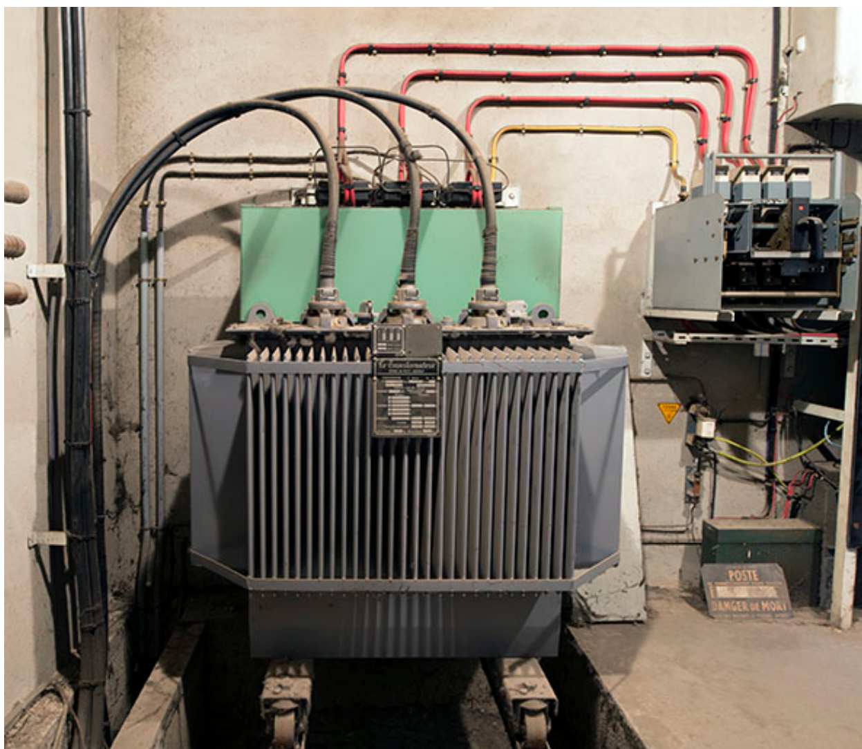
Transformateur 3 x 110 volts.
