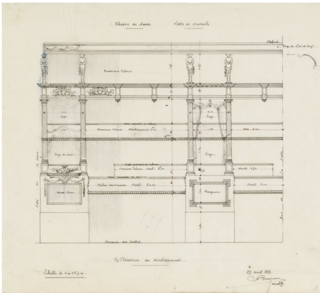
Théâtre de Nevers. Salle de spectacle. 1/2 Elévation du développement. 27 avril 1898.
