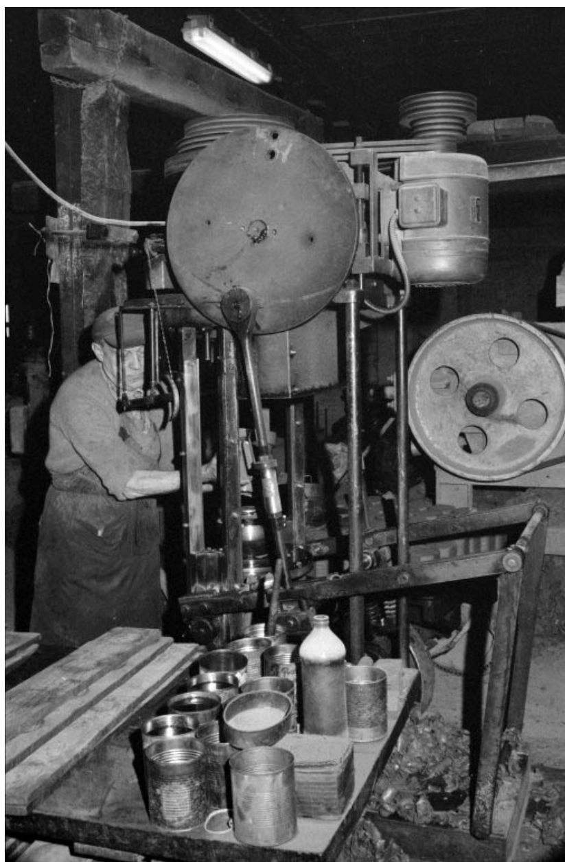
Poterie et briqueterie Martin, Etrepigny : mouleuse à pots de fleur Crochon.
