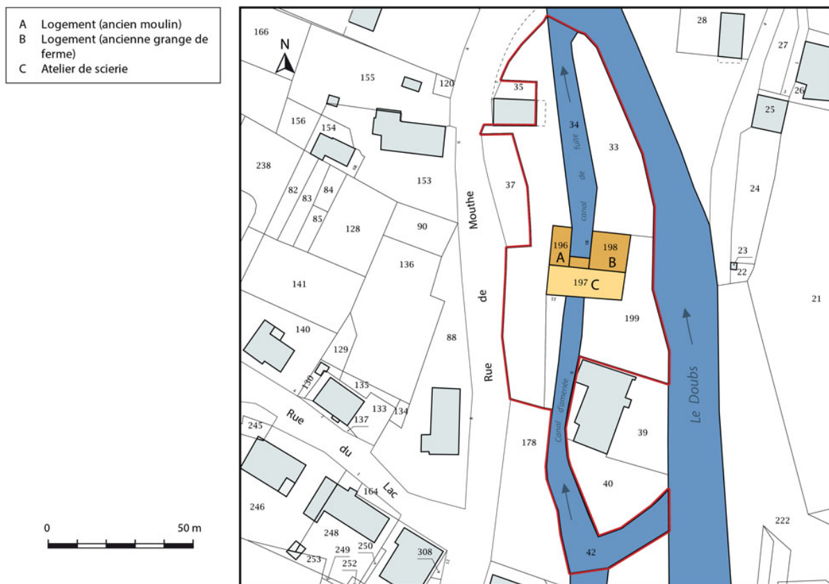
Plan-masse et de situation. Extrait du plan cadastral, 2016, section AC.
