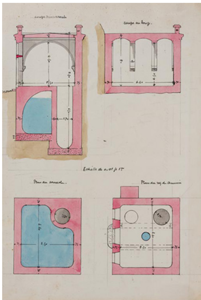
Bâtiment des machines (1895).
