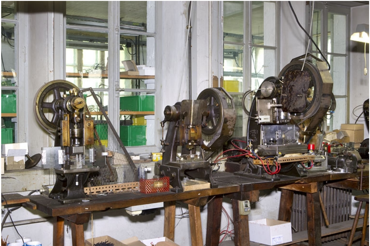
2e, 3e et 4e presses. De gauche à droite : presse Bréguet Frères, presse sans nom et presse Richert-Laval type Perla.
