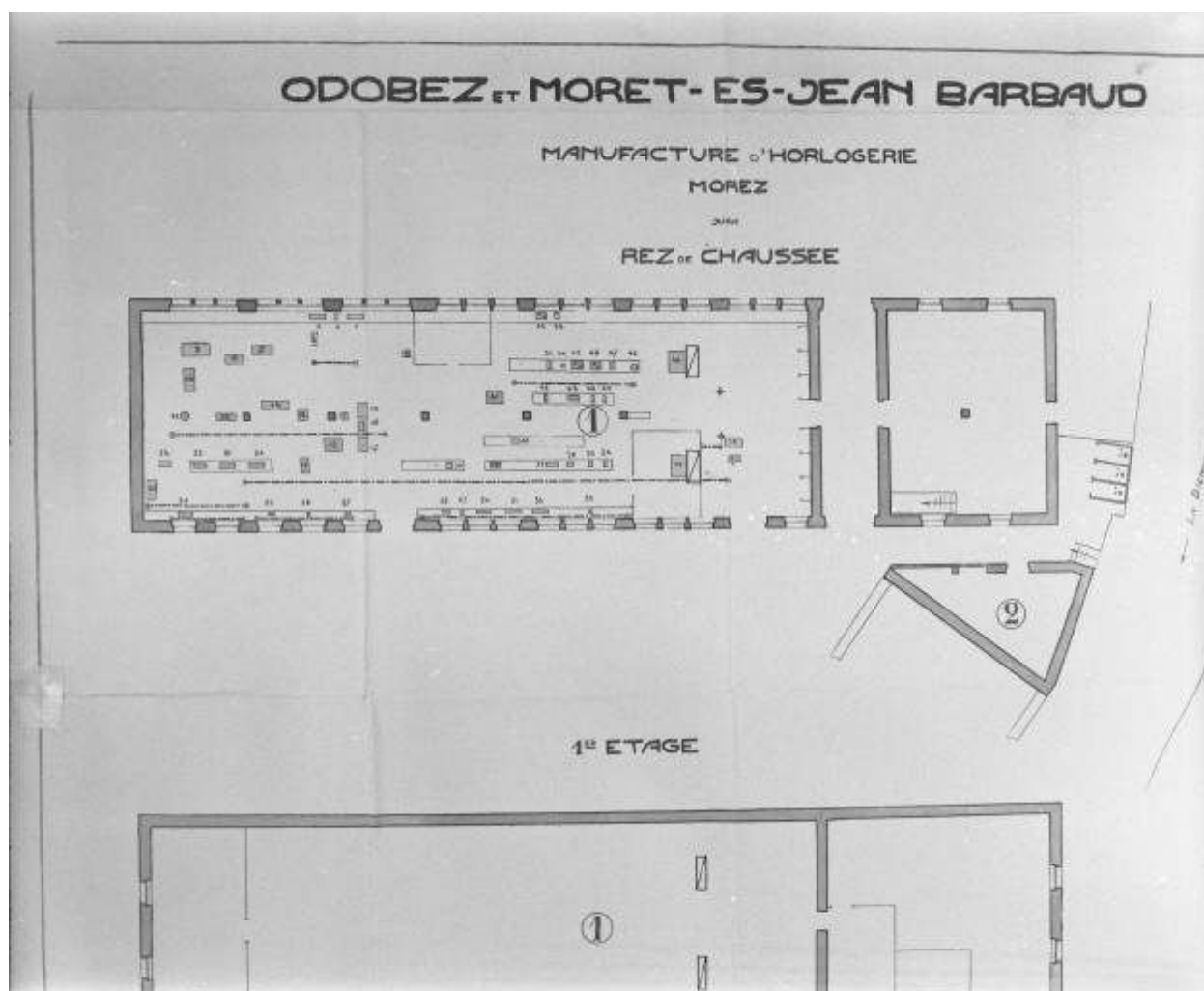
Odobet et Moret-ès-Jean-Barbaud. Manufacture d'horlogerie. Morez. [Détail du] Rez de chaussée. Dessin, 1927. Echelle 1:100.
