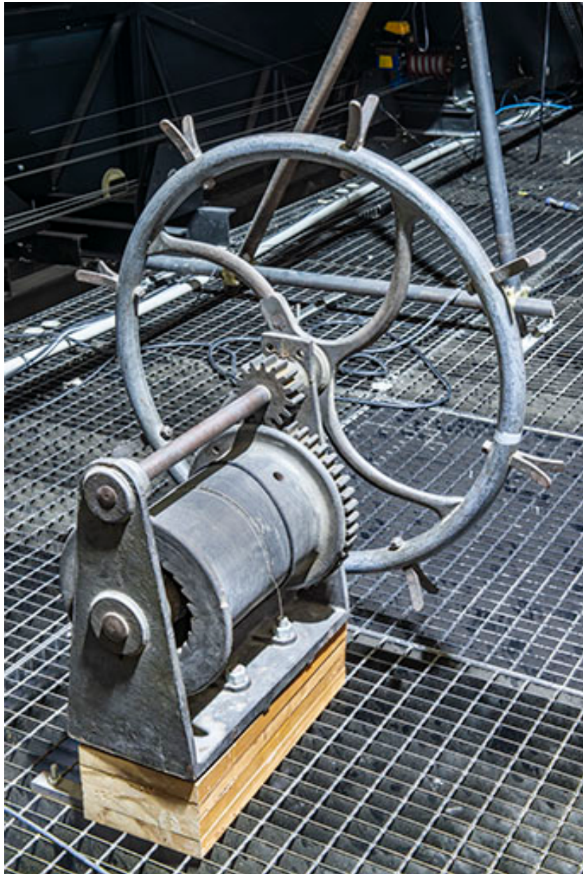
Treuil sur le gril de scène.
