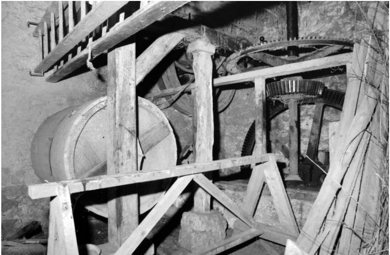
Tonneau de polissage et transmission.
