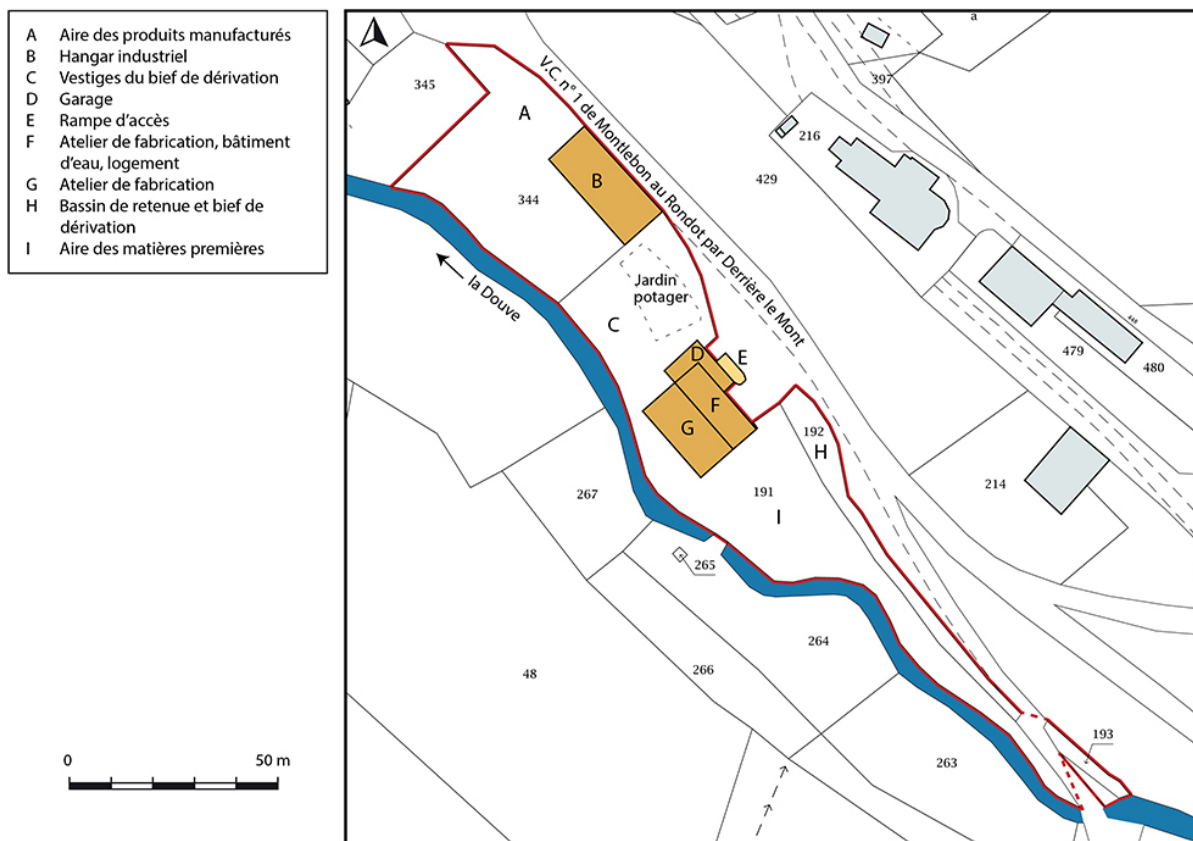
Plan-masse et de situation. Extrait du plan cadastral, 2016, section D, 1/1 000.
