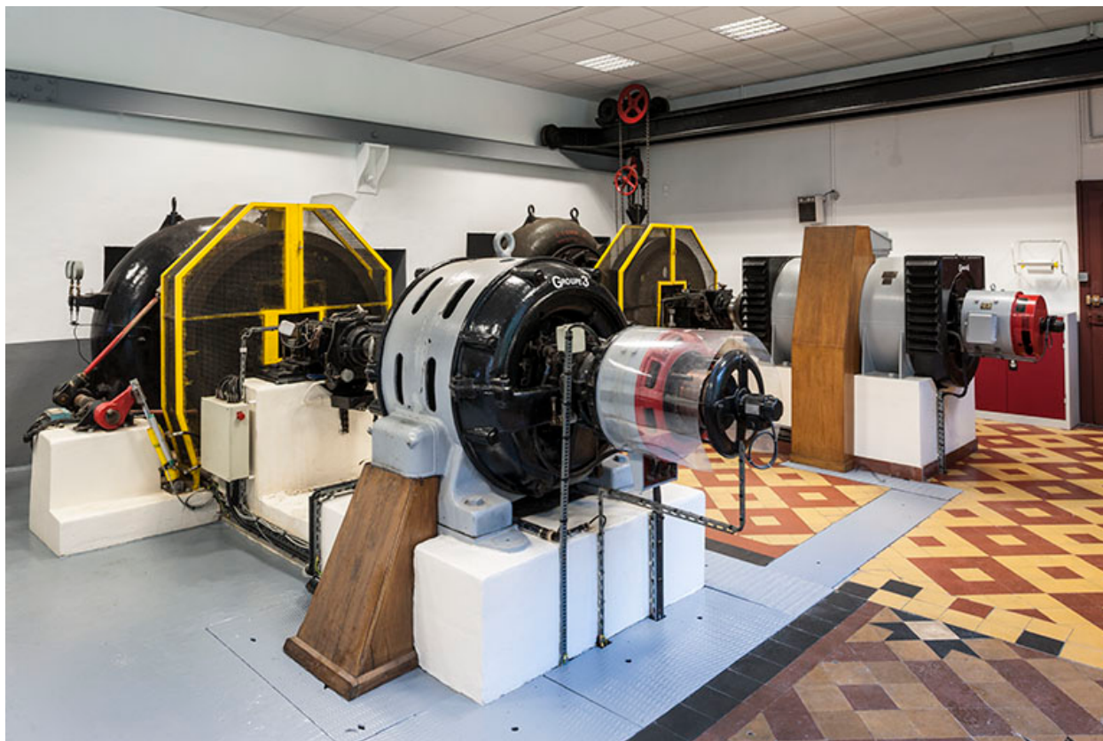
Groupes turbo-alternateurs en service.
