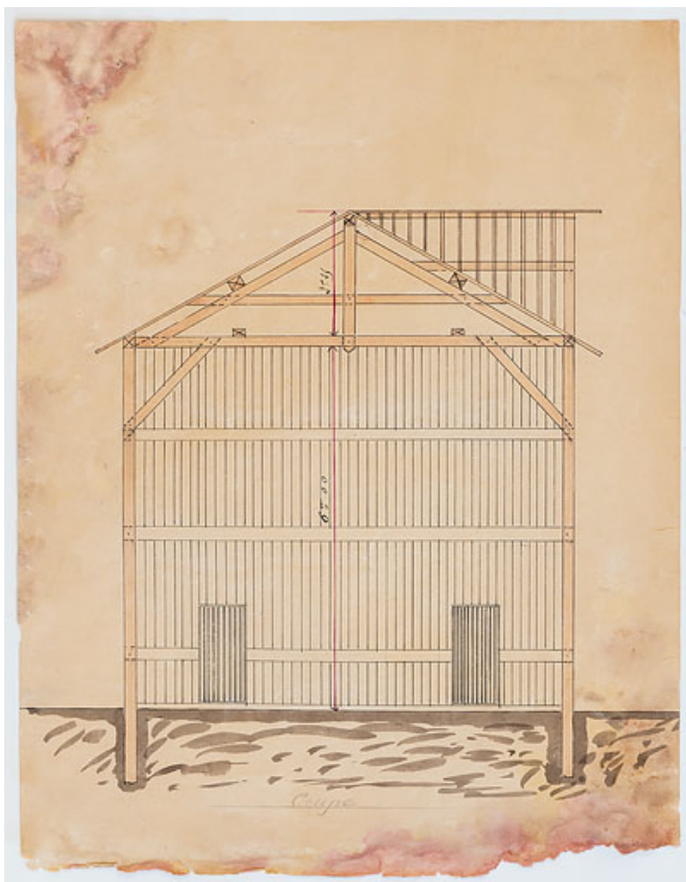
Projet de gymnase, coupe transversale.
