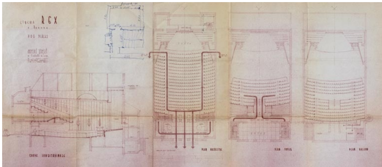
Cinéma Rex à Beaune. 800 places. Avant projet. 1er avril 1951.
