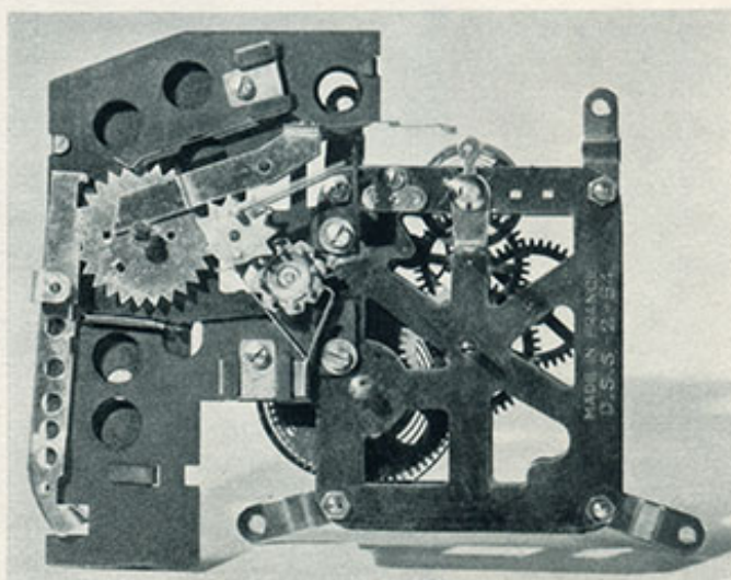
A GAUCHE DU MOUVEMENT D'HORLOGERIE, LE MÉCANISME A PRÉPAIEMENT DE LA PENDEULETTE CI-CONTRE.
