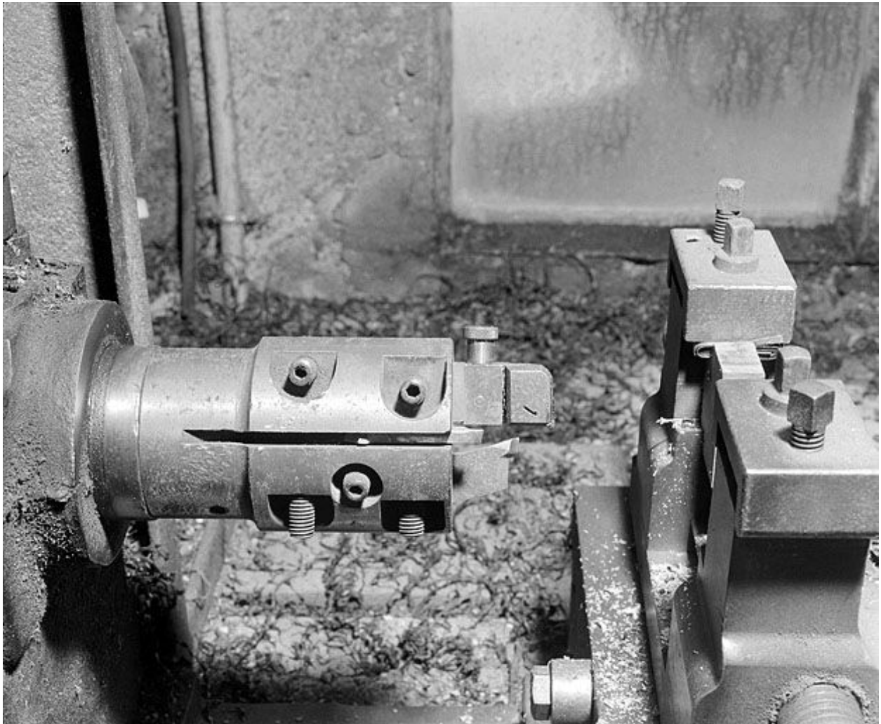
Détail du mandrin porte-outils (après rotation d'un quart de tour).
