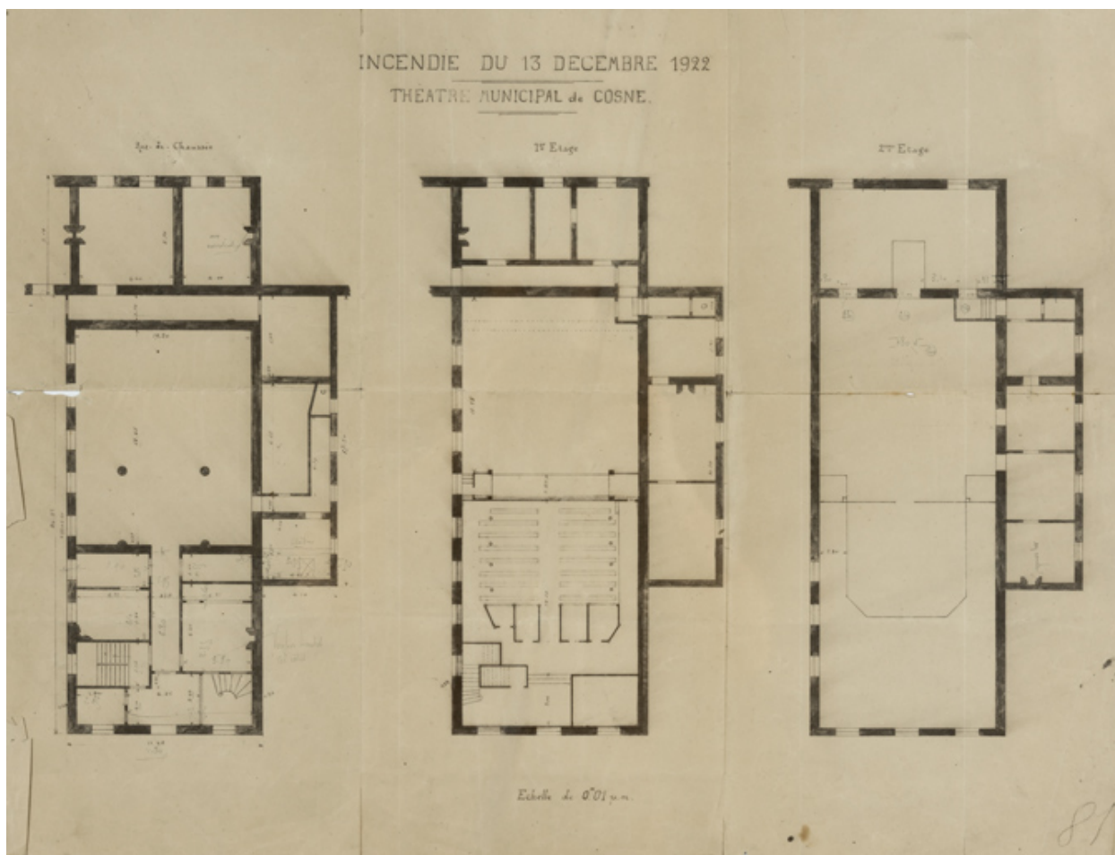
Incendie du 13 décembre 1922. Théâtre municipal de Cosne [plan du rez-de-chaussée et des deux étages]. S.d. [1922 ?].
