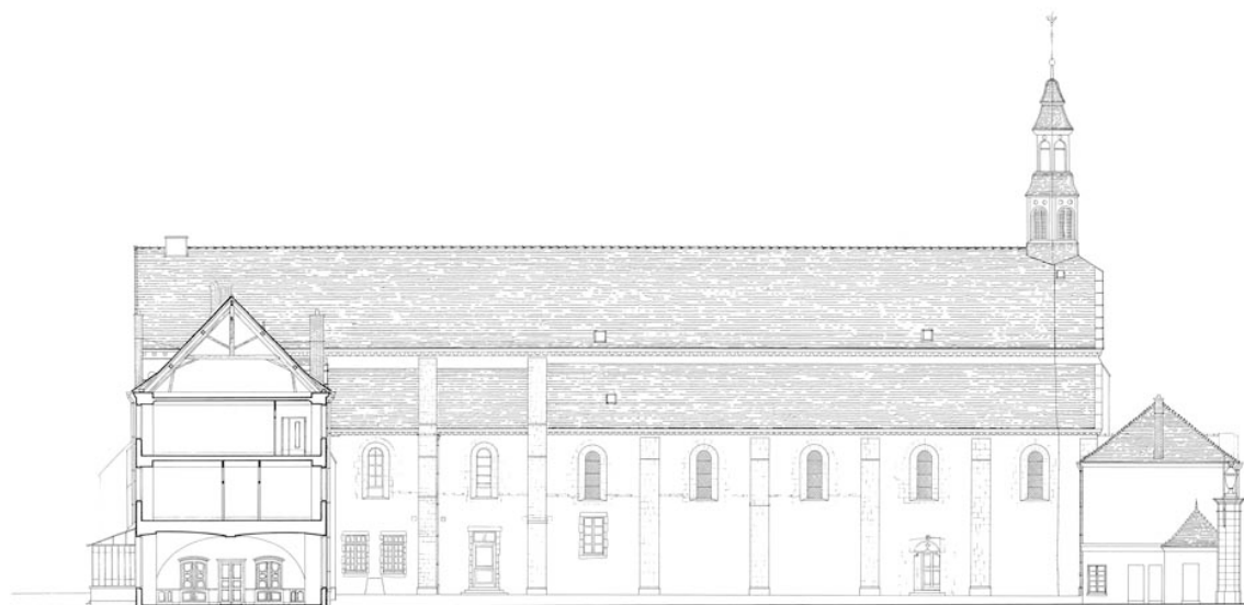
FACADE NORD SUR COUR
