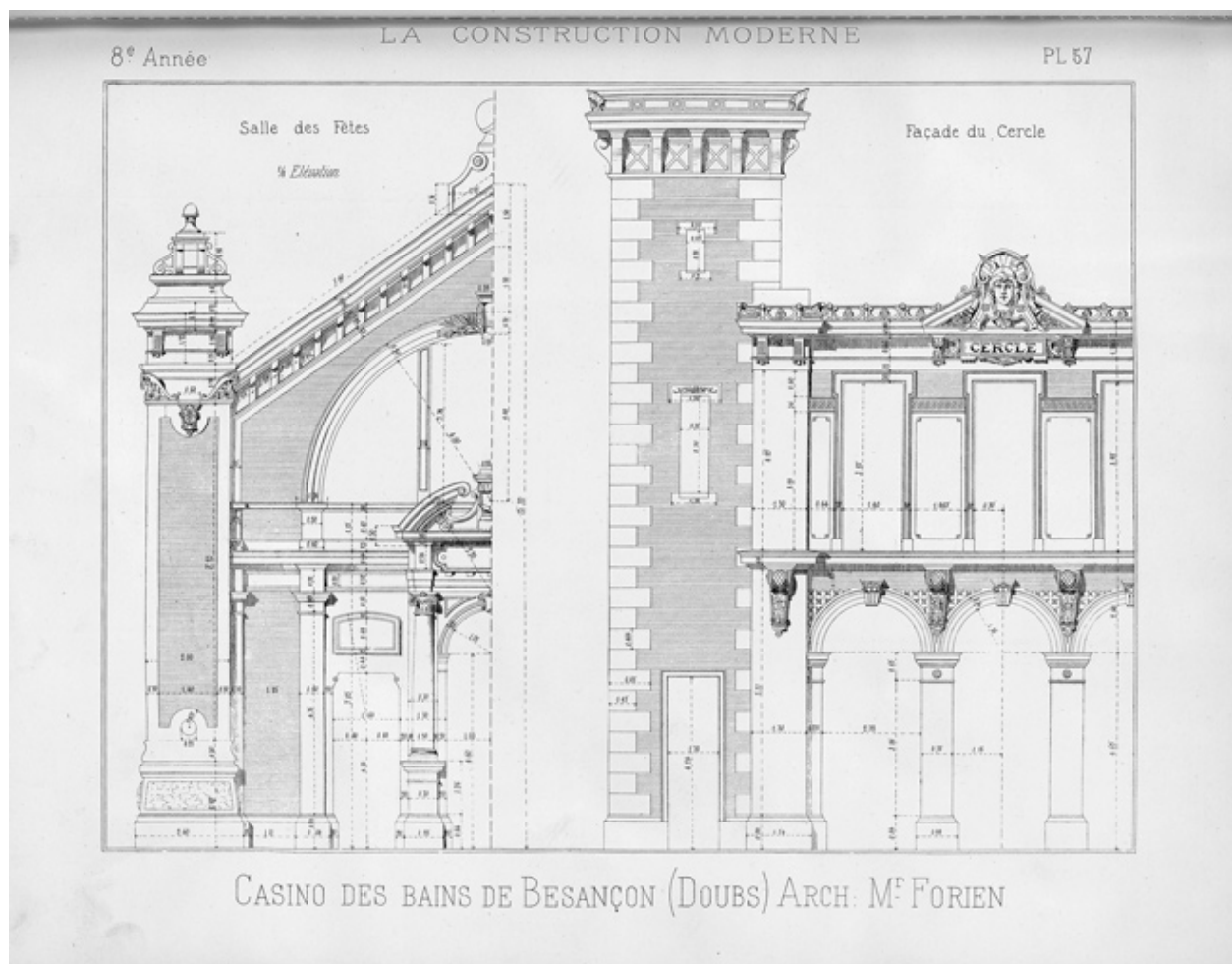
Élévation, détail (1893).
