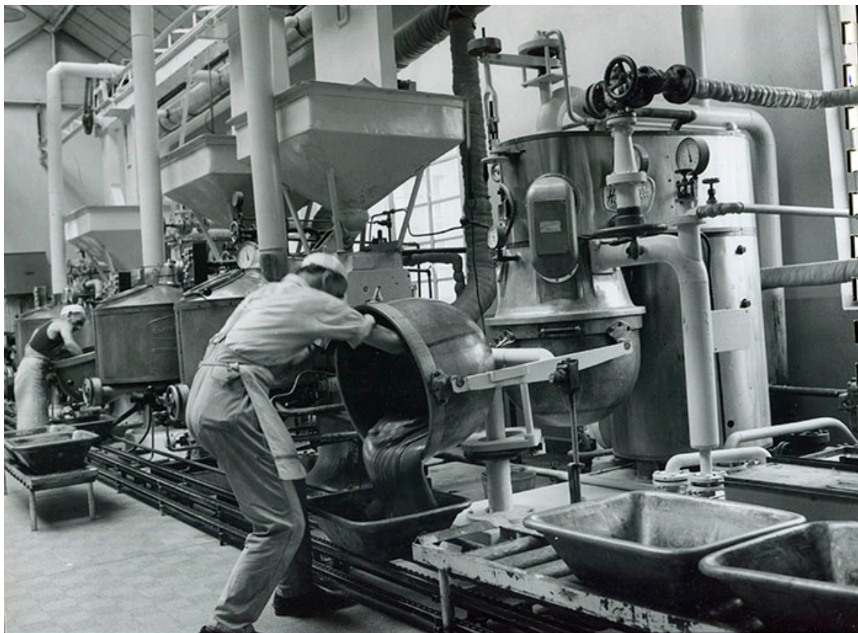
Cuiseurs continus et bassines à dissoudre, 1963.
