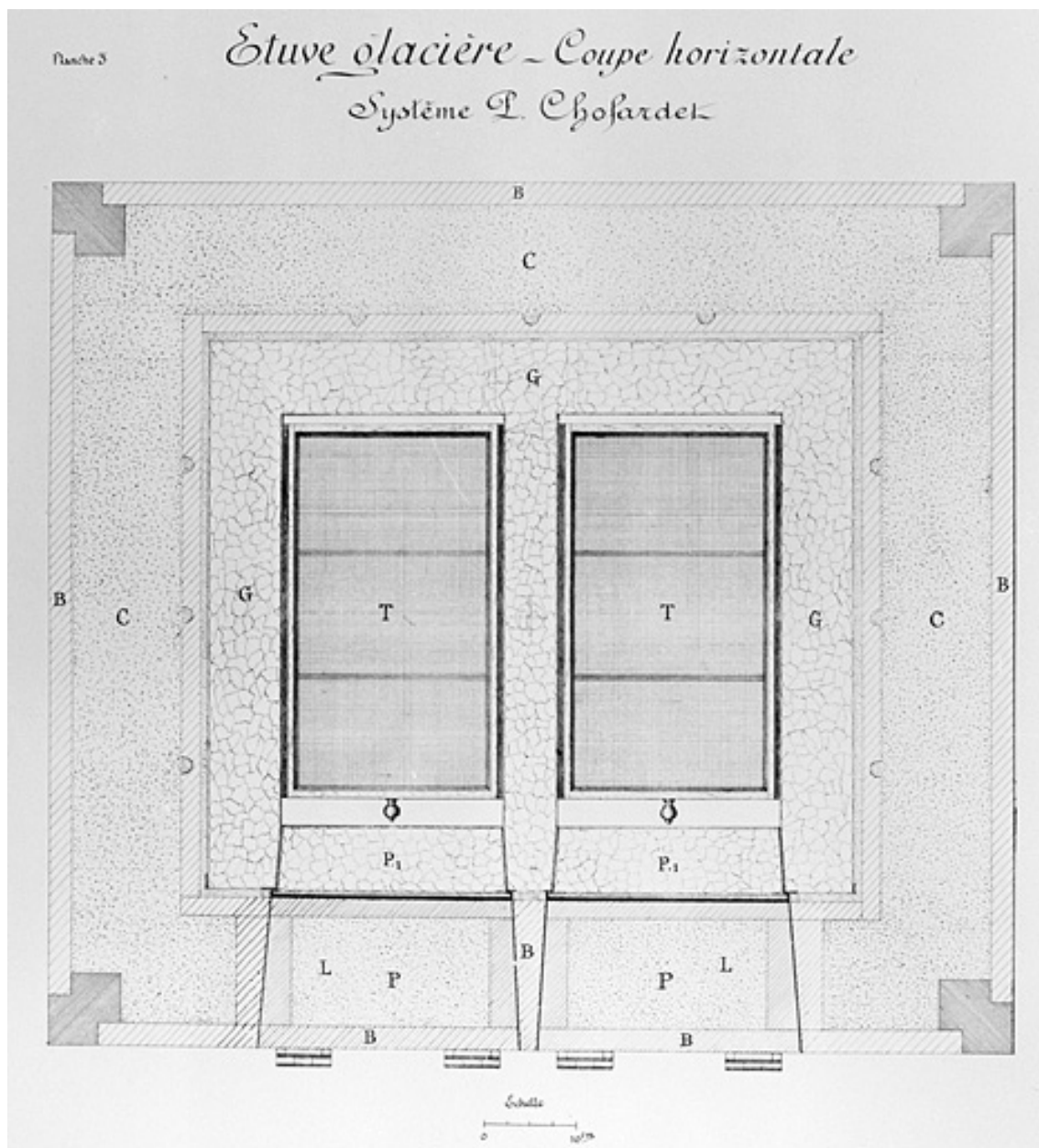
Etuve glacière système P. Chofardet. Coupe horizontale, 1906.
