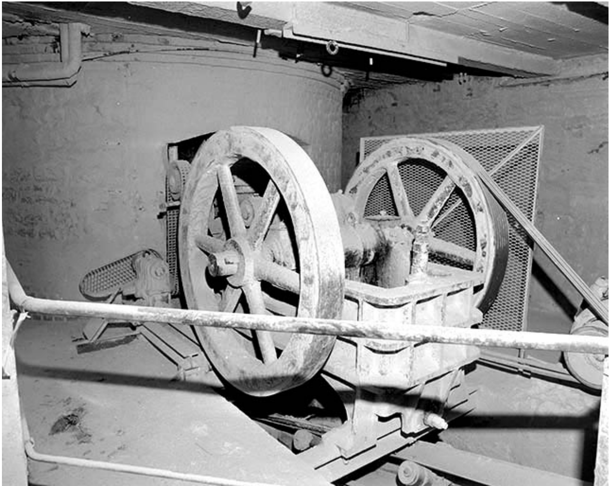
Concasseur à mâchoires : vue de trois quarts.
