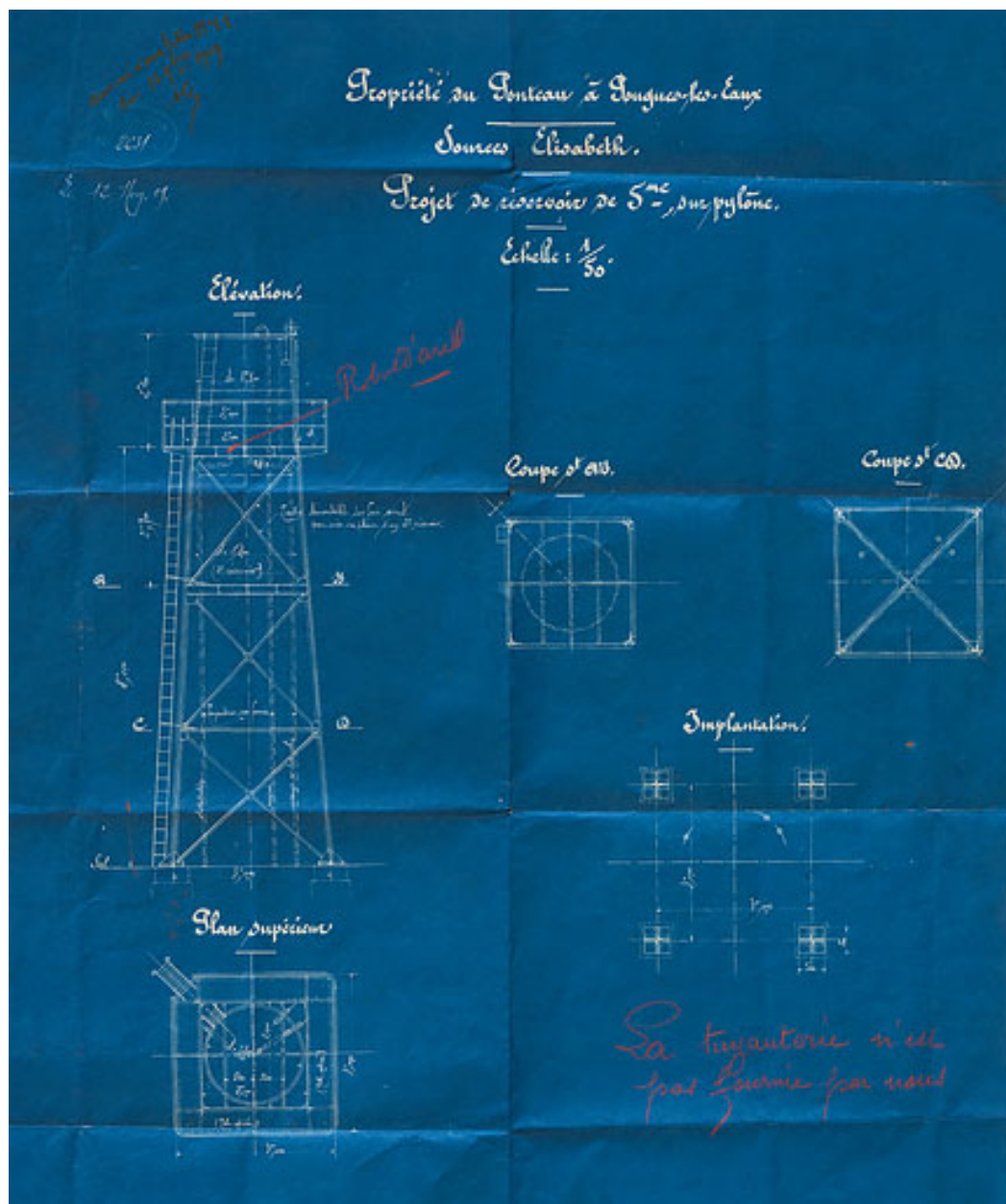
Plan et élévation du réservoir (1909).
