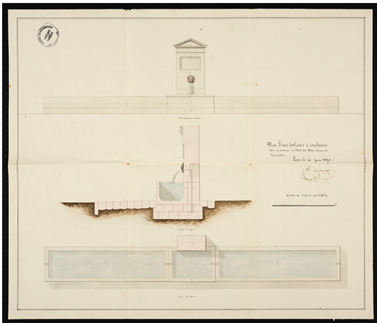
Plan d'une fontaine à construire (1829).
