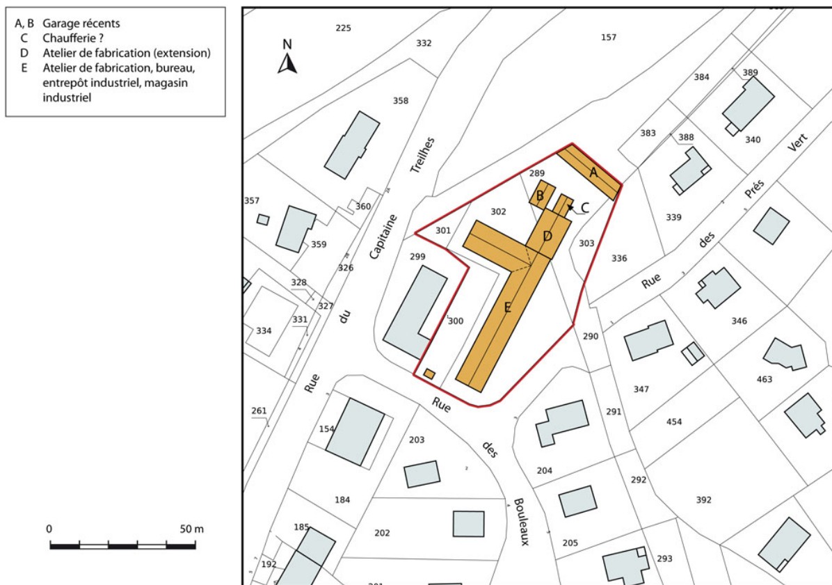
Plan-masse et de situation. Extrait du plan cadastral, 2014, section AB.
