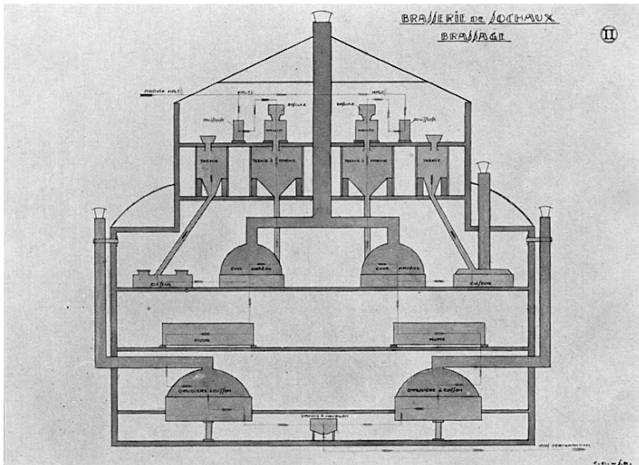
Coupe de la salle de brassage.
