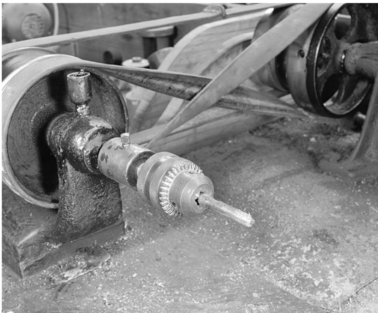
Détail du taraud.
