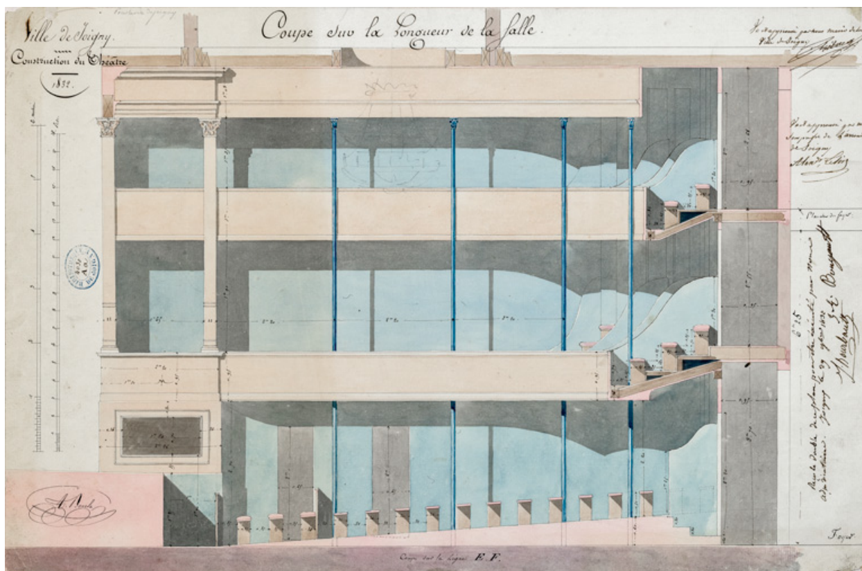
Construction de la salle de spectacle. Coupe sur la longueur de la salle. Pour la Ville de Joigny. 1832.
