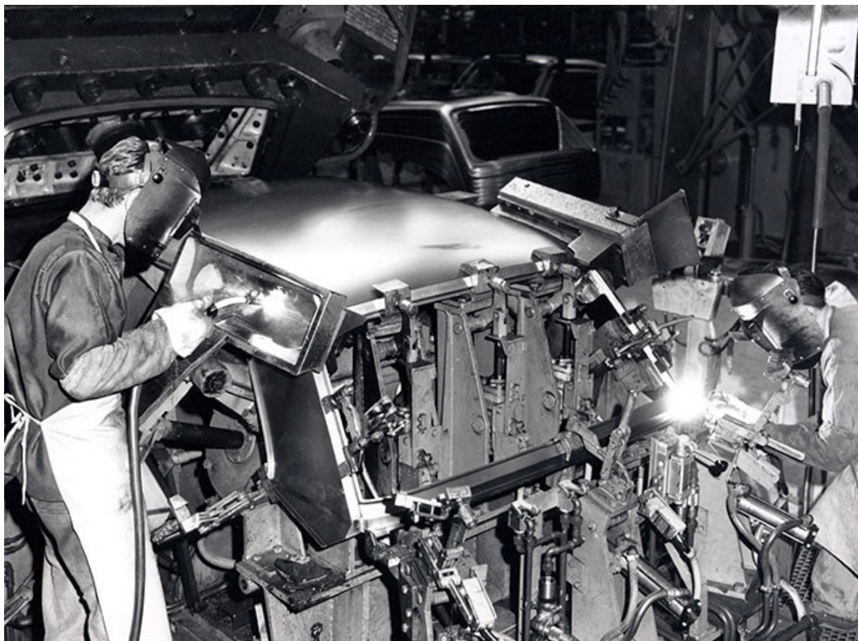
Automobile : assemblage par soudure de la caisse d'une automobile Peugeot, 30 septembre 1965.
